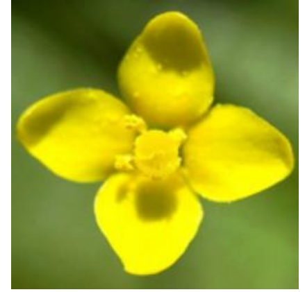
Cicendia filiformis
