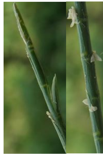
Hainardia cylindrica
