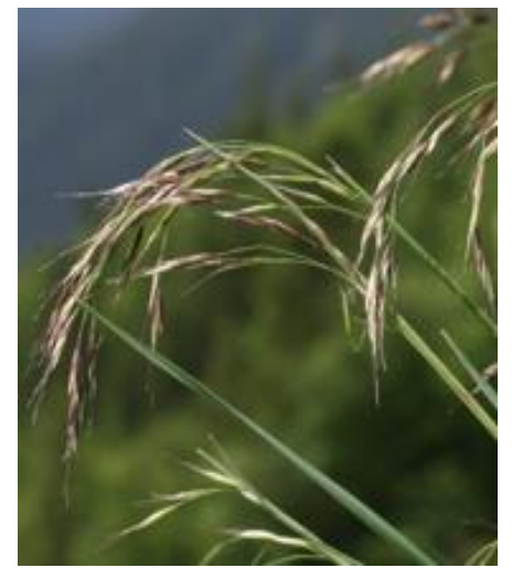
Helictotrichon parlatorei
