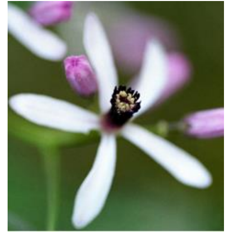
Melia azedarach
