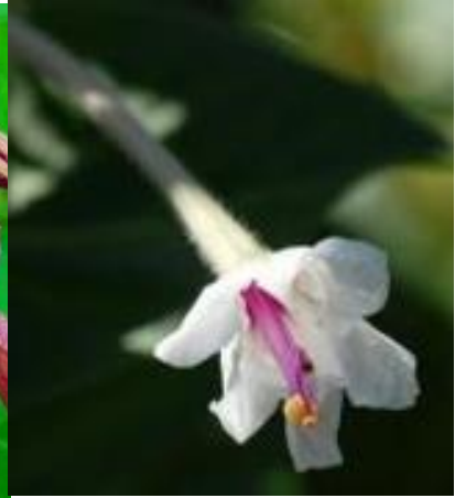
Mirabilis jalapa
