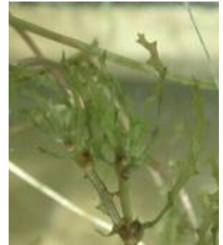
Najas marina
