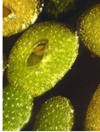
Wolffia arhiza
